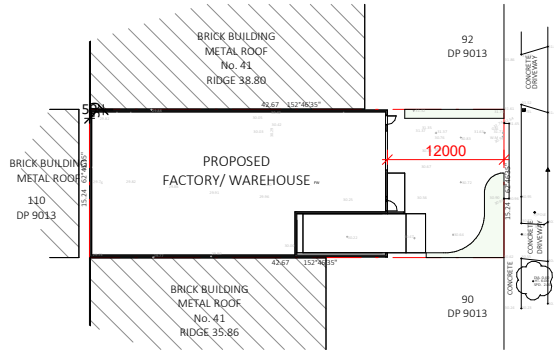
1 SITE PLAN - NP 1 : 500
